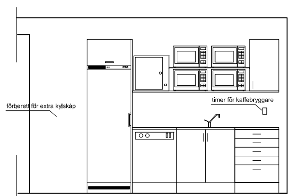
ELEVATION A-A KÖKSINREDE
